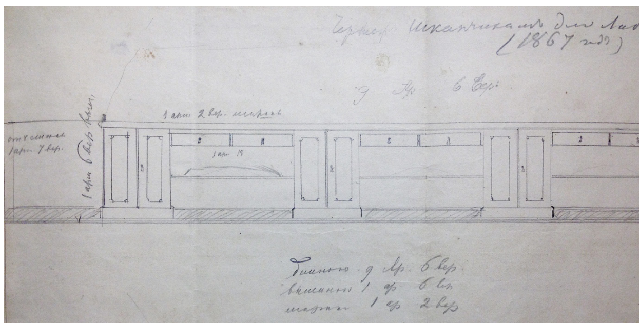
Рис. 4. Чертеж стола для химической лаборатории Института Корпуса инженеров путей сообщения. 1867 (Канцелярия института... 1867–1868). Публикуется впервые
