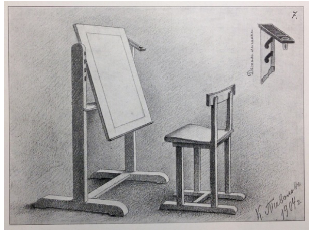
Рис. 12. Комплект из мольберта для рисования и стула. Рисунок К. Тиволовича. 1904 (Дело о выдаче пособий... 1903–1904). Публикуется впервые
