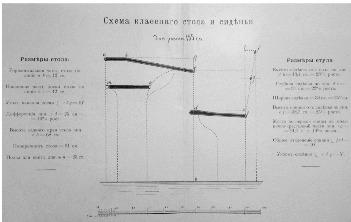
Рис. 8. Схема классного стола и сиденья для роста 155 см. 1904 (Дело о выдаче пособий... 1903–1904). Публикуется впервые
